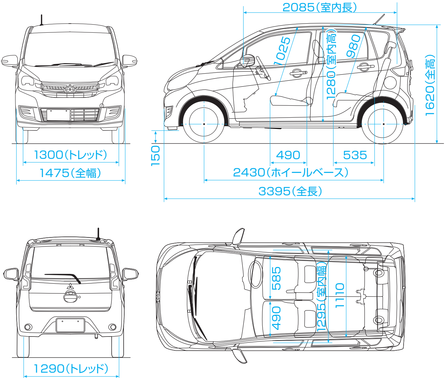
●eKワゴン 外観四面図(G 2WD) 単位 : mm
