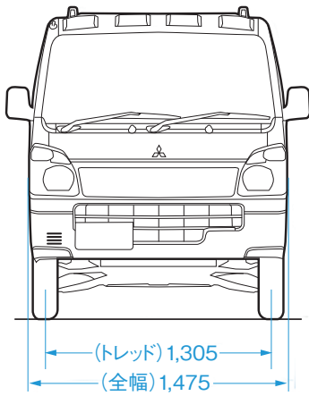
外観 4 面図 < M > 単位 : mm
