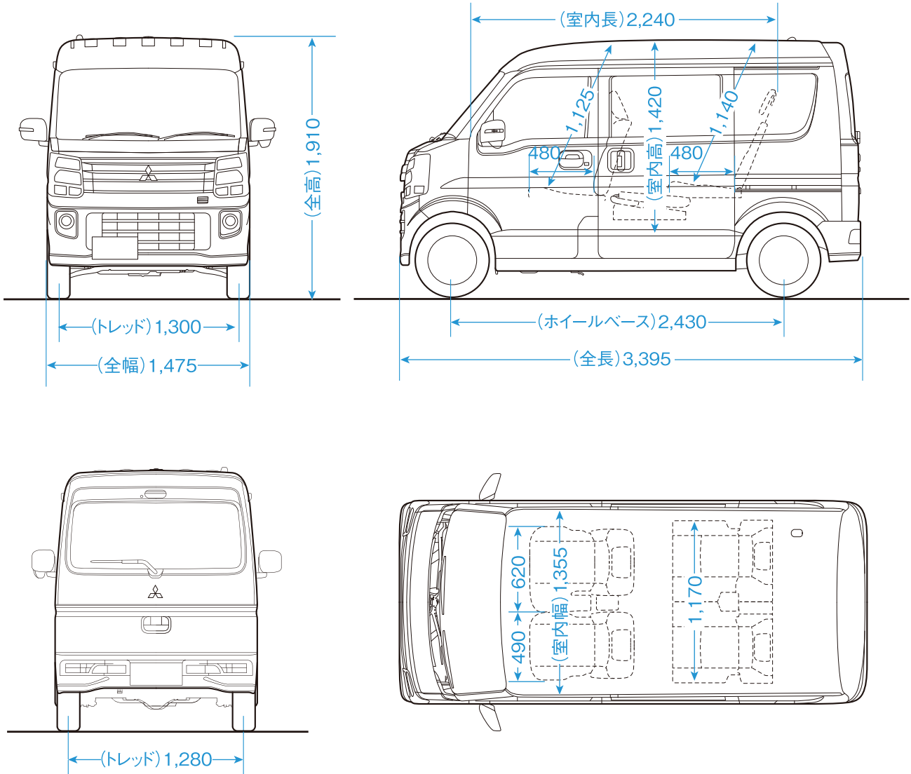
■ 外観 4 面図 < G スペシャル > 単位 : mm
