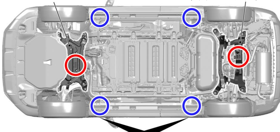
<ジャッキ>
