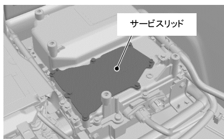
↓ 車両前方
